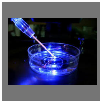
MTT Assay
